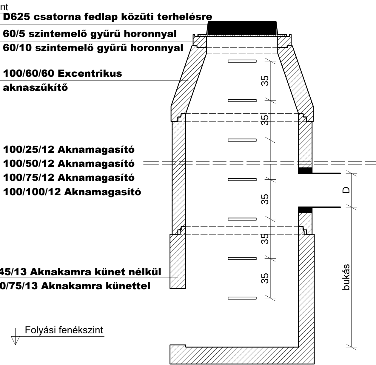
B-B metszet
