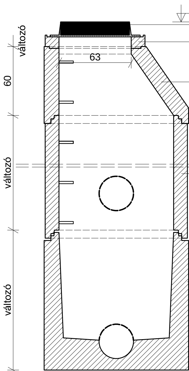
A-A metszet
