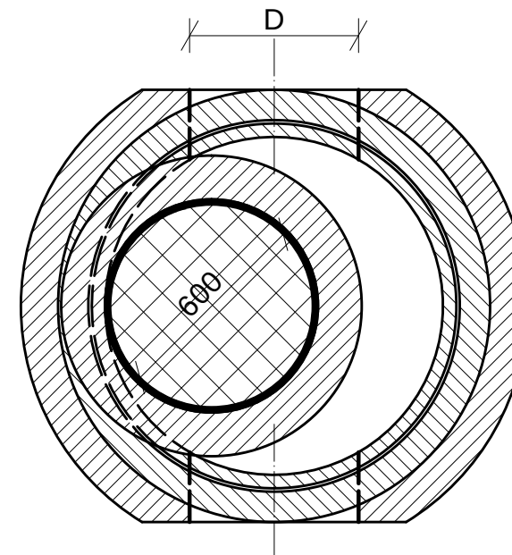
Felülnézet
