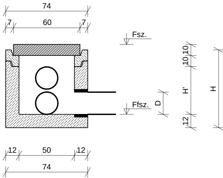
Metszet
