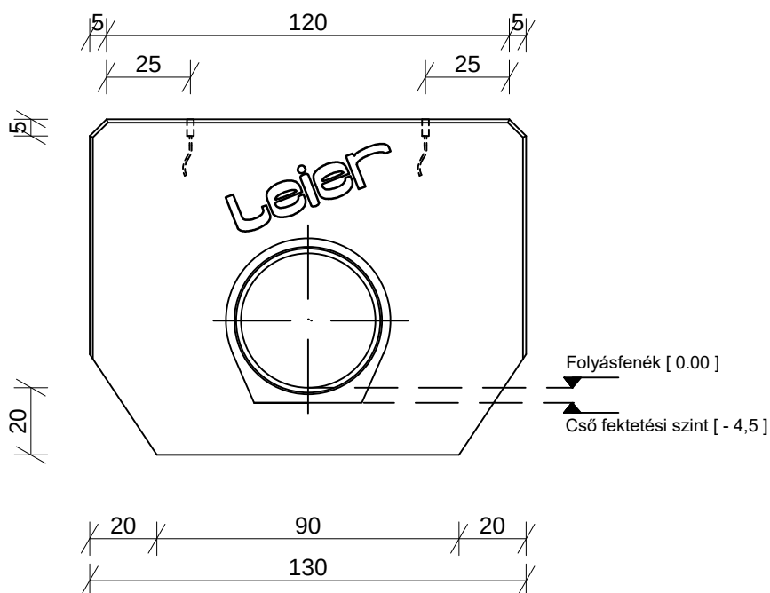
ELŐLNÉZET
